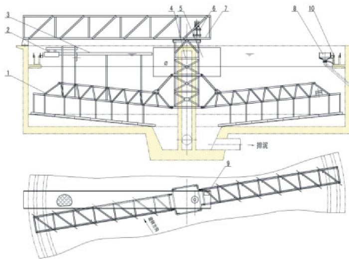
1、刮泥桁架 2、浮渣耙板 3、浮渣刮板 4、中心架 5、稳流筒 6、动力驱动装置 7、行走平台 8、浮渣漏斗 9、电气控制装置 10、溢流装置
